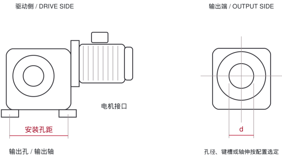
蜗杆与蜗轮轴线交错；空心输出接口与电机法兰分别确认 安装接口示意 · 轮廓不按比例 · 具体数值见对应型号表 / INTERFACE GUIDE — NOT TO SCALE
