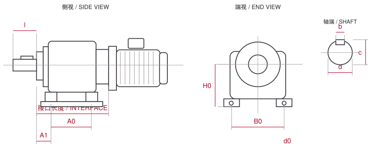
H0 中心高 · A0 / B0 孔距 · d0 孔径 · d / I 轴径与轴伸 安装接口示意 · 轮廓不按比例 · 具体数值见对应型号表 / INTERFACE GUIDE — NOT TO SCALE
