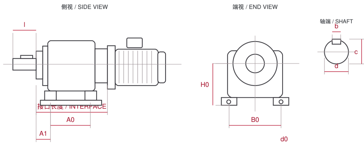
H0 中心高 · A0 / B0 孔距 · d0 孔径 · d / l 轴径与轴伸 安装接口示意 · 轮廓不按比例 · 具体数值见对应型号表 / INTERFACE GUIDE — NOT TO SCALE
