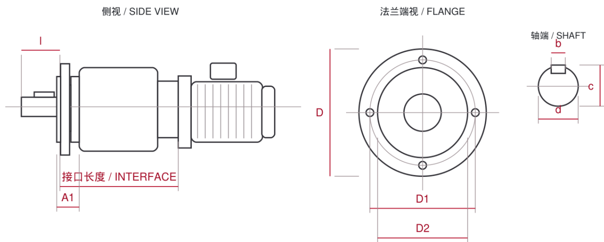
D 法兰外径 · D1 孔中心圆 · D2 止口 · d0 孔径 · d / I 轴径与轴伸 安装接口示意 · 轮廓不按比例 · 具体数值见对应型号表 / INTERFACE GUIDE — NOT TO SCALE
