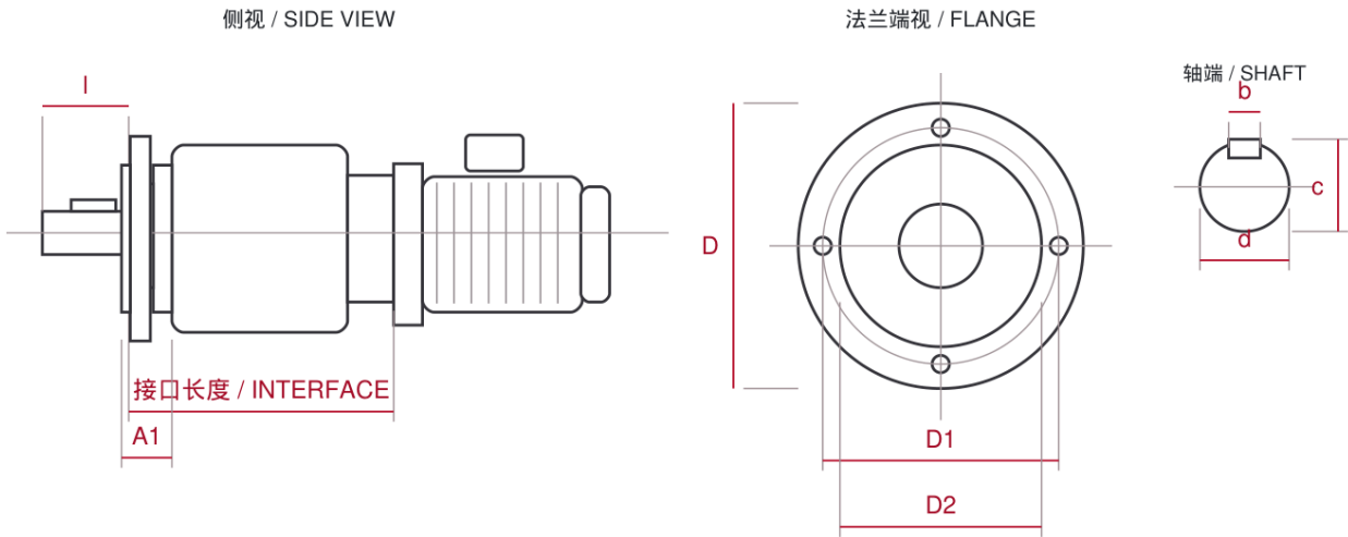
D 法兰外径 · D1 孔中心圆 · D2 止口 · d0 孔径 · d / l 轴径与轴伸
