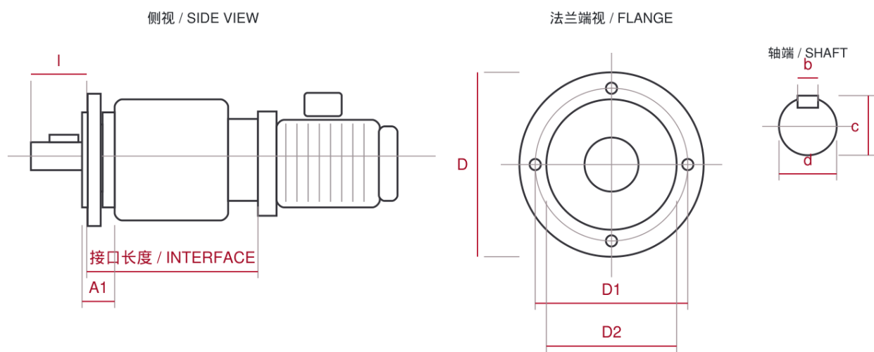
D 法兰外径 · D1 孔中心圆 · D2 止口 · d0 孔径 · d / l 轴径与轴伸 安装接口示意 · 轮廓不按比例 · 具体数值见对应型号表 / INTERFACE GUIDE — NOT TO SCALE
